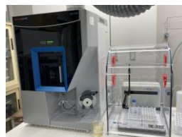
ICP 発光分析装置 (サーモフィッシャー・サイエンティフィック製 iCAP PRO XP Duo)
