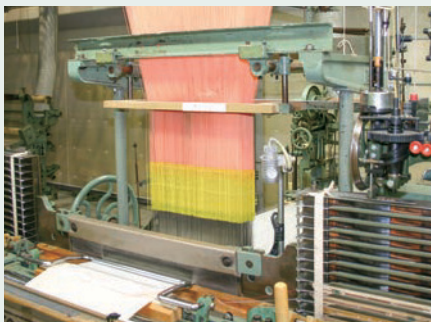
▲ ストーブリ社製電子ジャカードを搭載したシャトル織機
